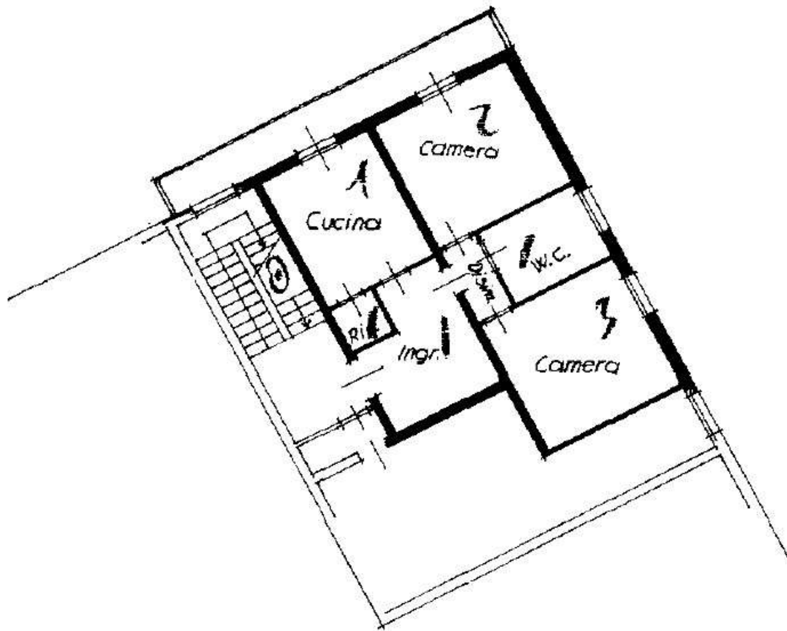
PIANO PRIMO H. 3,00
